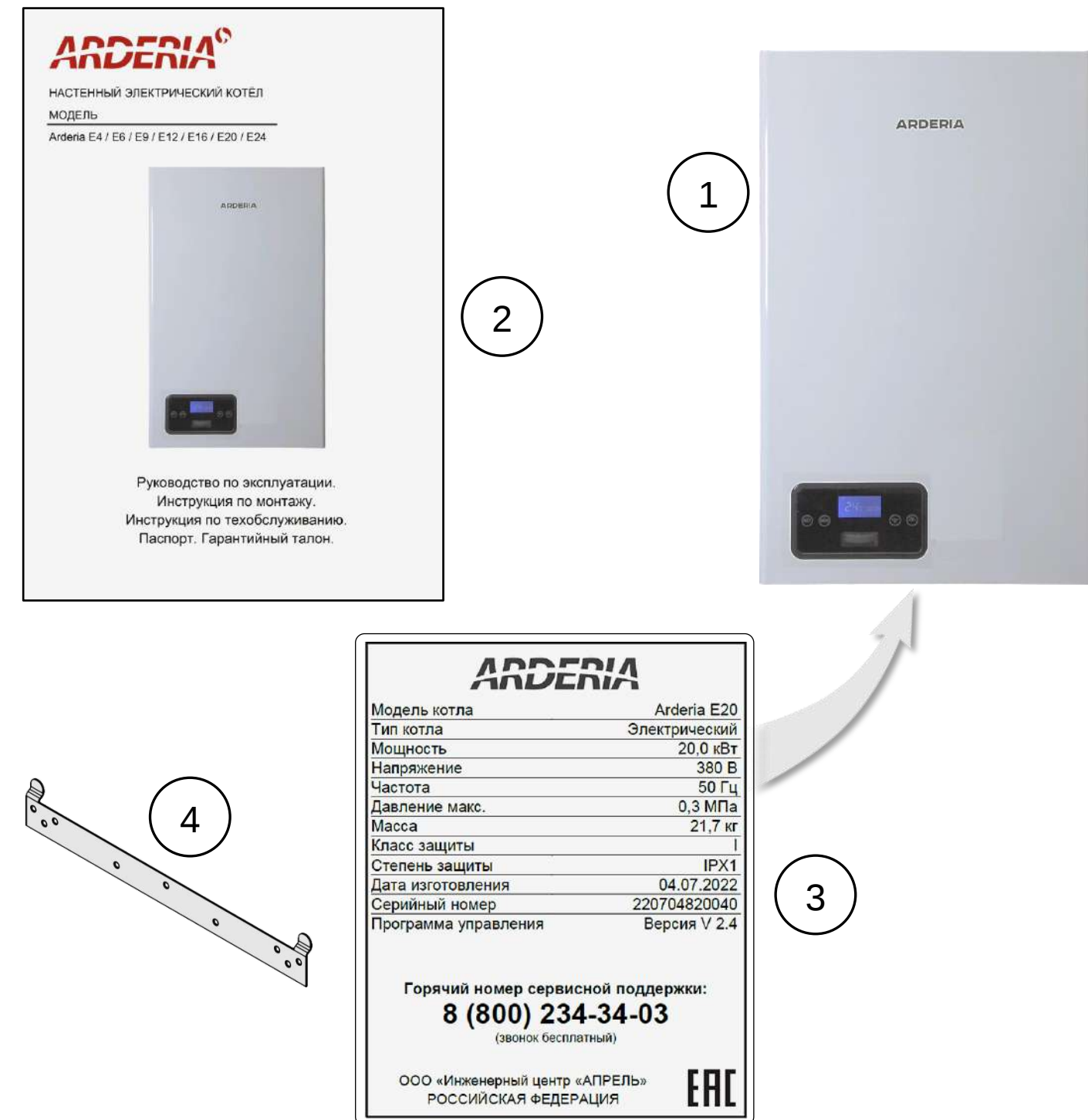
Рис. 4 Комплект поставки
