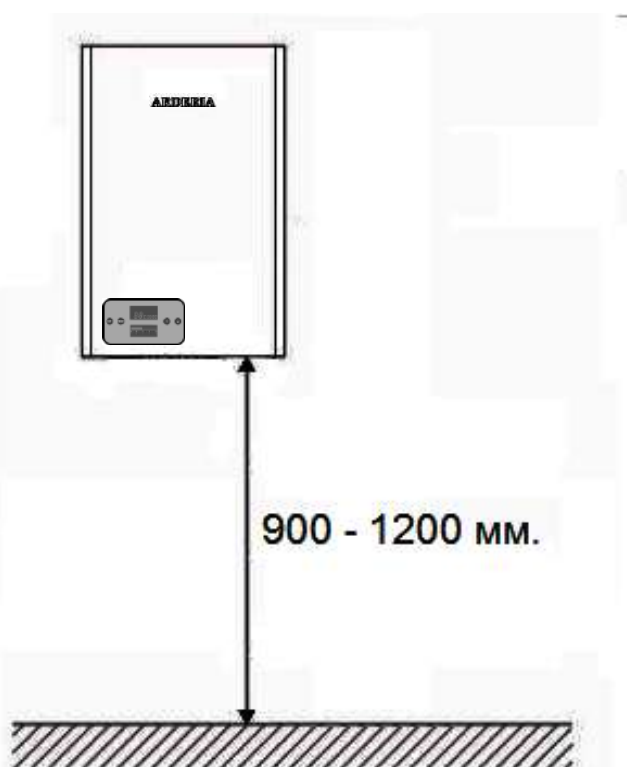
Рис. 10 Монтажные расстояния
