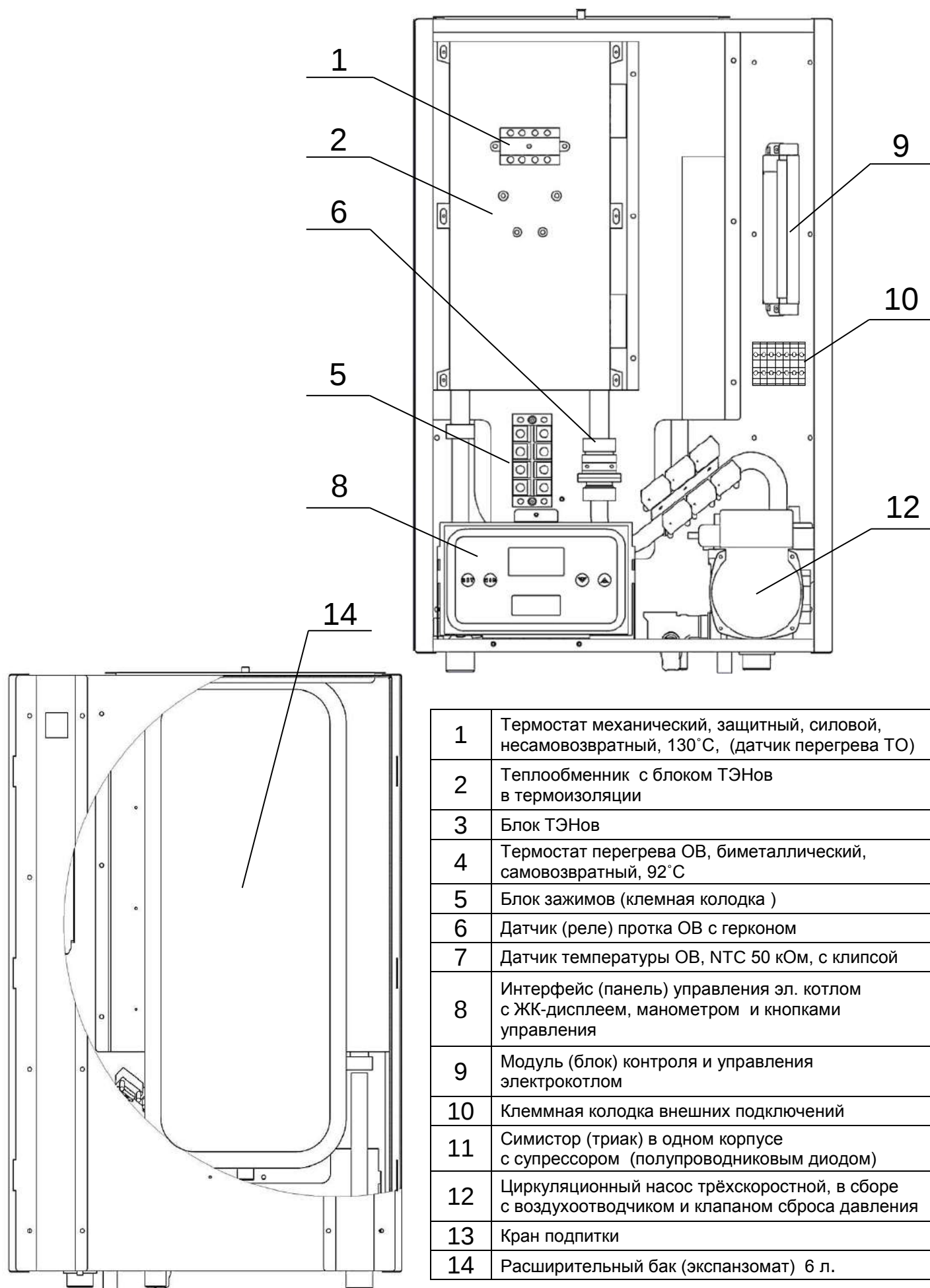
Рис. 2 Внутренне устройство
