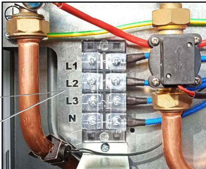
Рис. 14 Трёхфазное подключение
